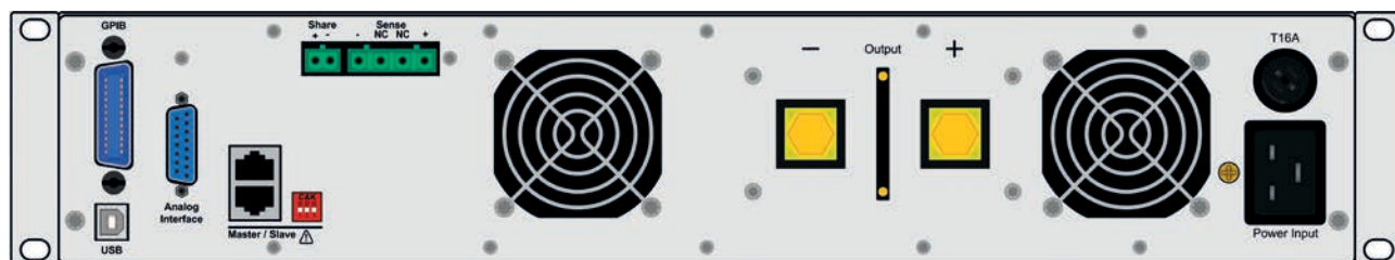
Vue arrière avec l'option 3W
