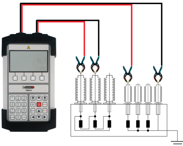
Raccordement de TWR-H à un transformateur de distribution triphasé
