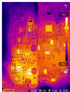
Cartes de circuit imprimé
