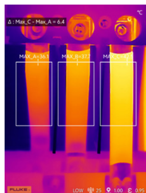
Calcul automatique de la différence de température triphasée
