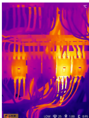
Armoires de distribution électrique
