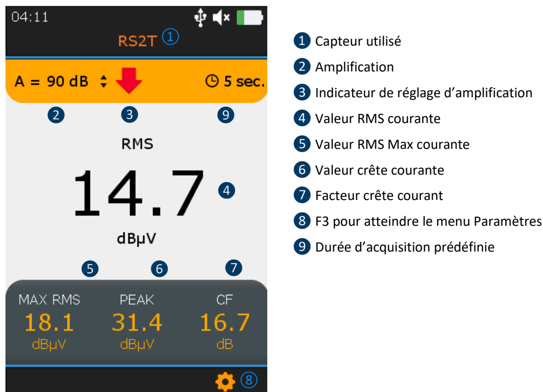
Figure 10-1 Écran de mesure ultrasonore
