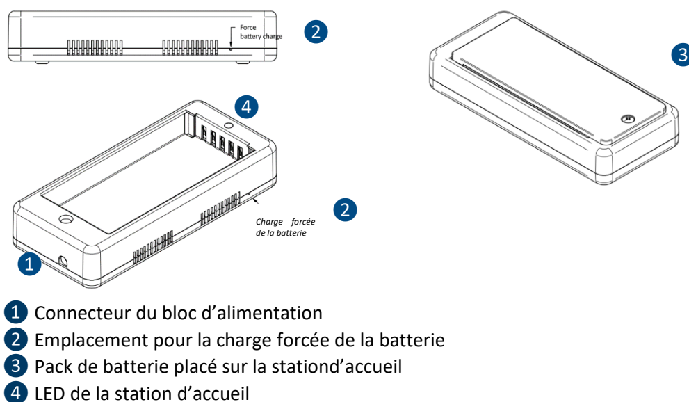
Figure 6-1 Recharge de la batterie
