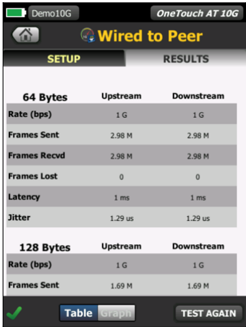
Figure 12. Analyse détaillée de connexions filaires jusqu'à l'équipement pair
