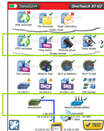
Figure 1. L'autotest réalise une mesure complète des performances du réseau depuis le point de vue de l'utilisateur final, du câble aux services et aux applications (les résultats de test obtenus avec le OneTouch AT doté du module G2 pour les réseaux filaires et Wi-Fi sont présentés)
