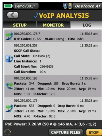
Figure 18. L'analyse VoIP décrit le processus complet de configuration des appels ainsi que la qualité de l'appel dans chaque direction
