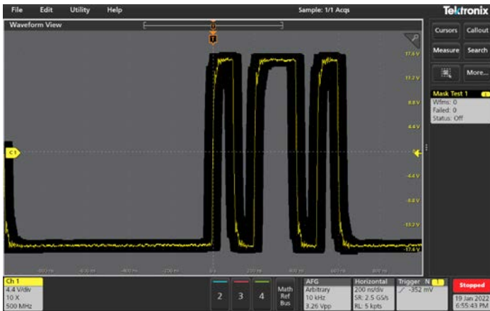
Test de limite de masque basé sur le signal de référence idéal
