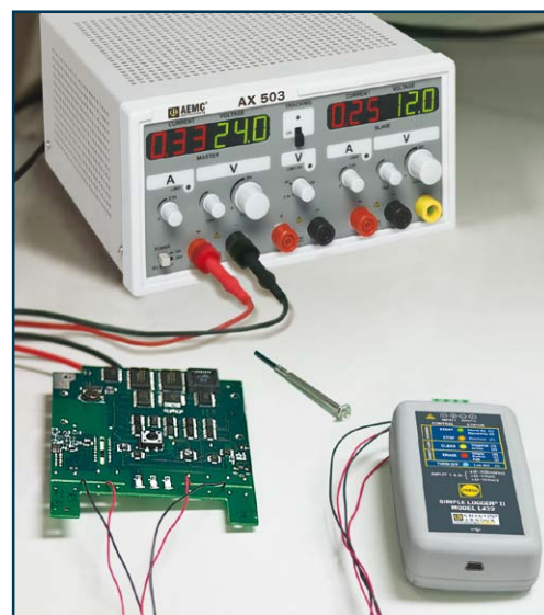
Enregistrement de deux sources de tension DC avec le modèle L432.
