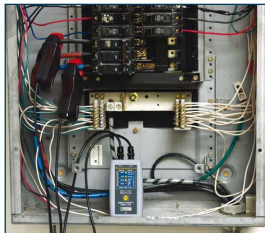
Enregistrement de deux phases sur le circuit d'alimentation du primaire avec le L102.
