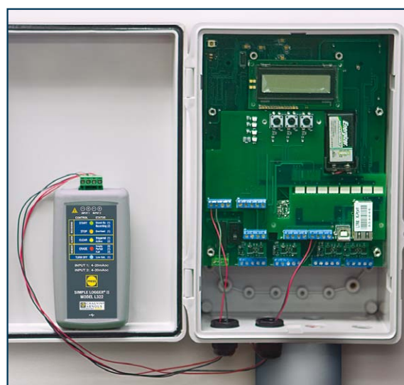
L322 enregistre un courant de boucle sur un tableau de contrôle de débit.
