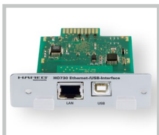
Interface Ethernet/USB pour applications indus- trielles H0730 (en option)
