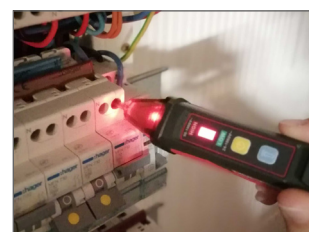
Indication visuelle et sonore de présence de tension
