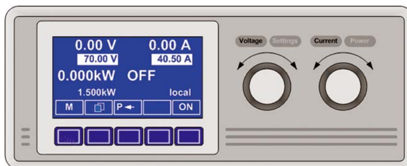
Drehgeber für Einstellungen Rotary knobs for settings
