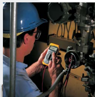
◀ FLUKE-719 Calibrateur de pression avec pompe électrique intégrée
