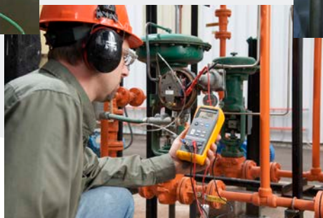
◀ FLUKE-719 Calibrateur de pression avec pompe électrique intégrée
