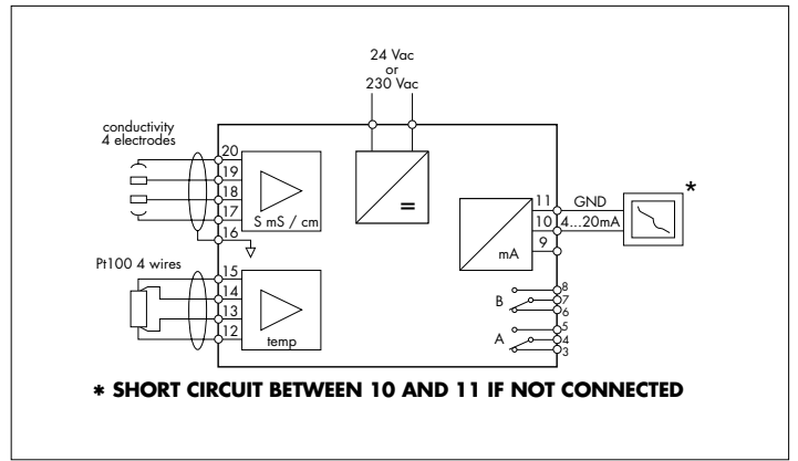
Fig.1 Transmetteur actif.
