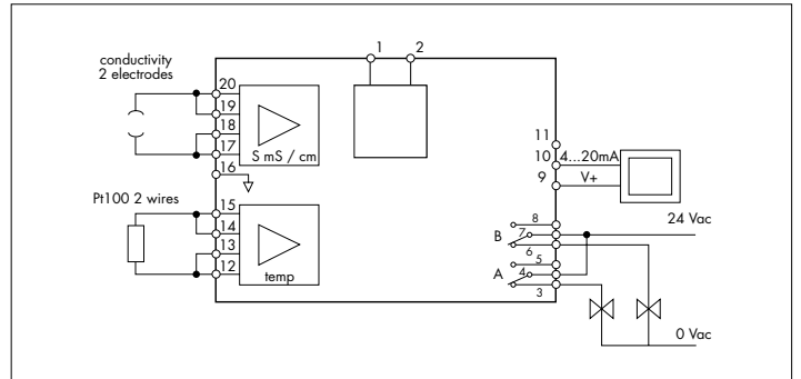
Fig.2 Transmetteur passif.
