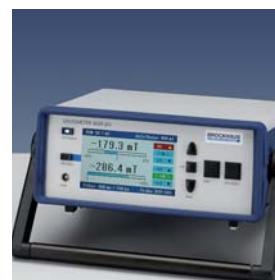
Gaussmeter BGM 201
