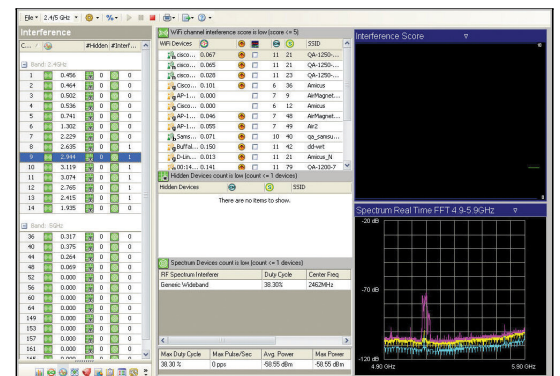
Figure 13: Analyse des interférences Wi-Fi et non Wi-Fi
