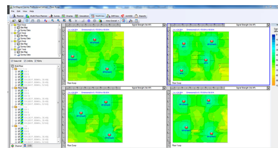
Figure 11: Déploiements multi-étage
