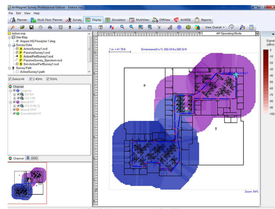
Figure 8: Carte thermique 802.11n
