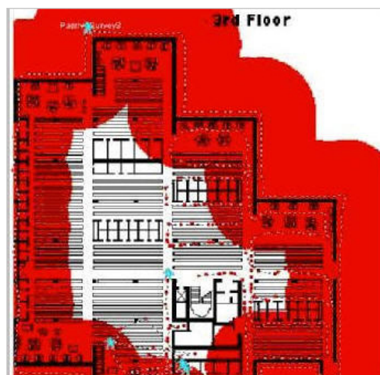
Figure 7: Débordement des radiofréquences à l'extérieur des locaux de l'entreprise
