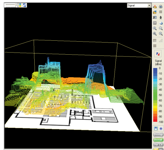
Figure 3: Affichage 3D permettant une visualisation des niveaux de signaux maximum/minimum
