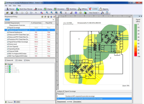
Figure 12: AirWISE pour l'analyse de sites
