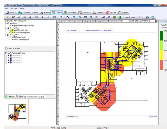
Figure 9: Schéma de couverture qualitatif des appels vocaux
