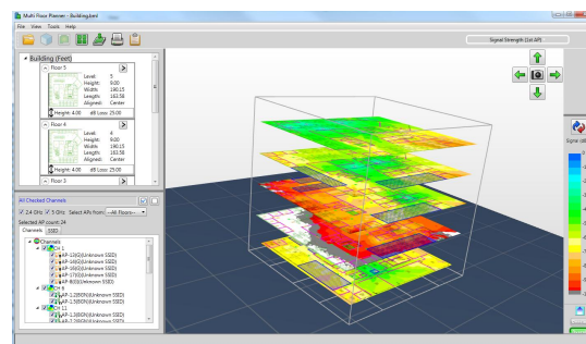
Figure 15: Modélisation sans fil automatisée avec AirMagnet Planner
