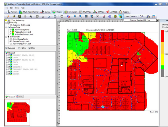
Figure 1 : Atténuez l'interférence de canal en visualisant la superposition primaire et secondaire de canaux
