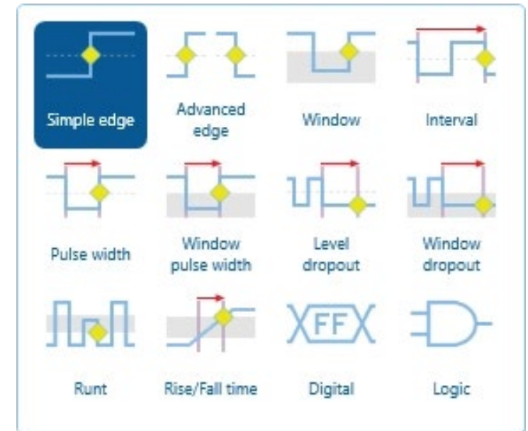
Sélection de déclenchement de déclencheurs avancés
